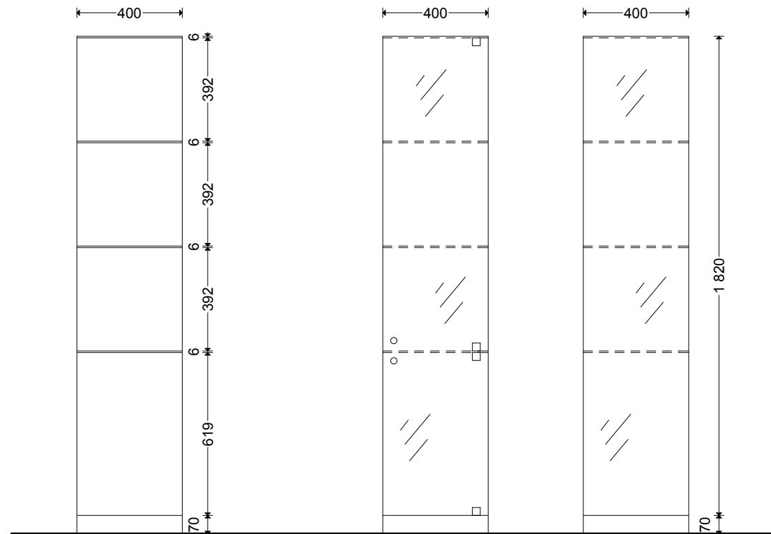
REZ M 1:20
