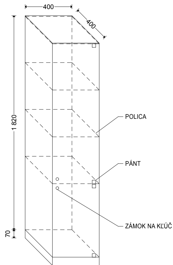
AXONOMETRIA
